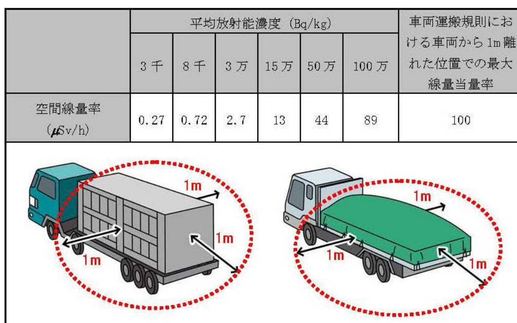
図 2.1.3-9 輸送車両から 1m の地点における空間線量率の試算例
