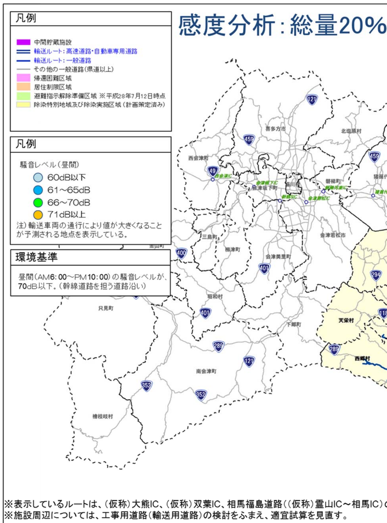
図 2.5.1-23 【感度分析：輸送量 20%増】本格輸送時「③生活：騒音（昼間）」の試算結果
