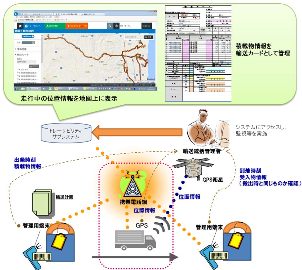
図 2.2.5-1 輸送車両の管理機能の概要
